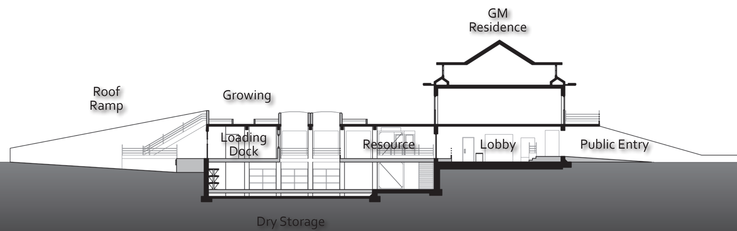
Section DD
