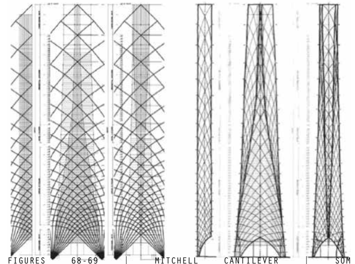
FIGURES 68-69 | MITCHELL | CANTILEVER | SOM
