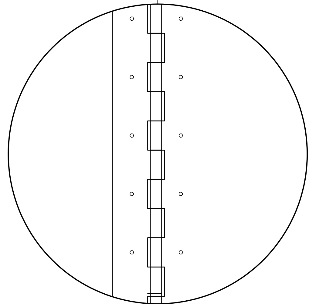
PIANO HINGE SCALE: 6" = 1'-0"
