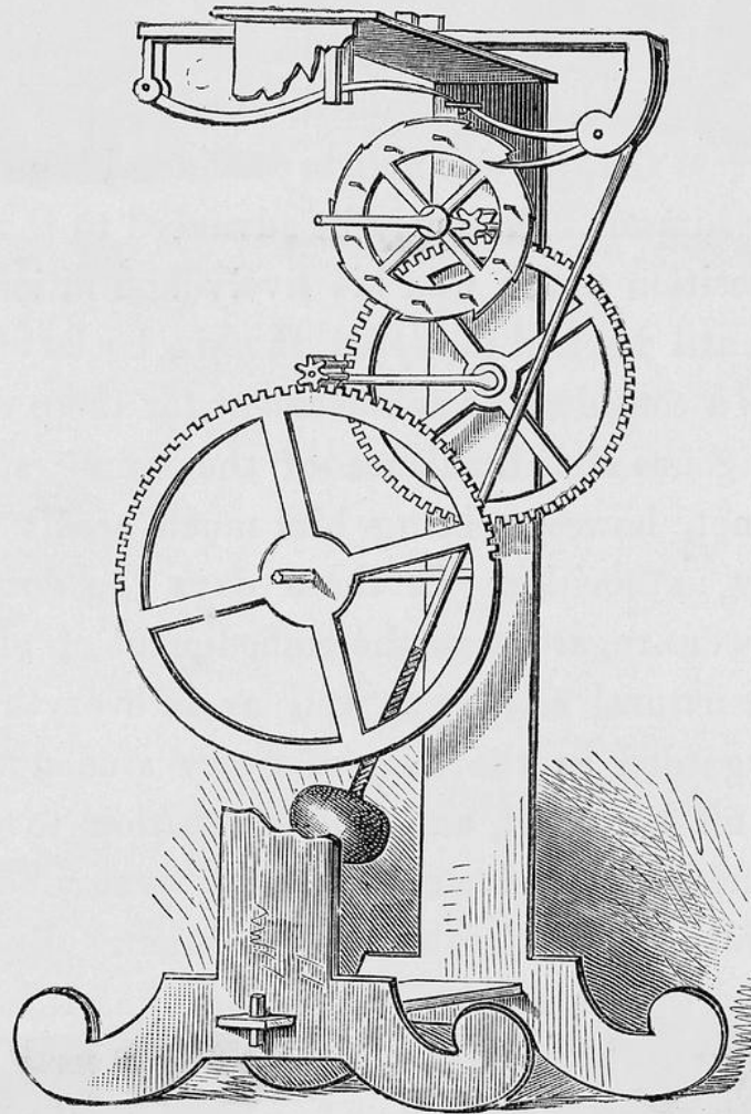
Galileo's Pendulum.
